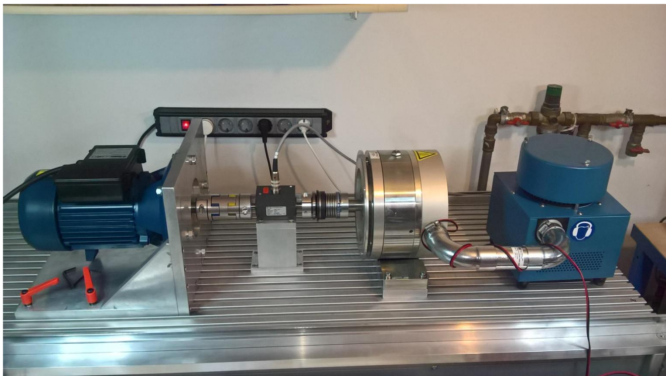
Antriebskette aus Motorhalter, Kupplungen, Drehmomentaufnehmer und Hysteresenbremse mit Luftkühler
